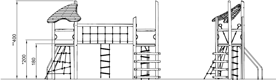
NRO2002 1:100
